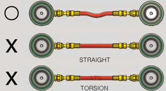
TORSION
